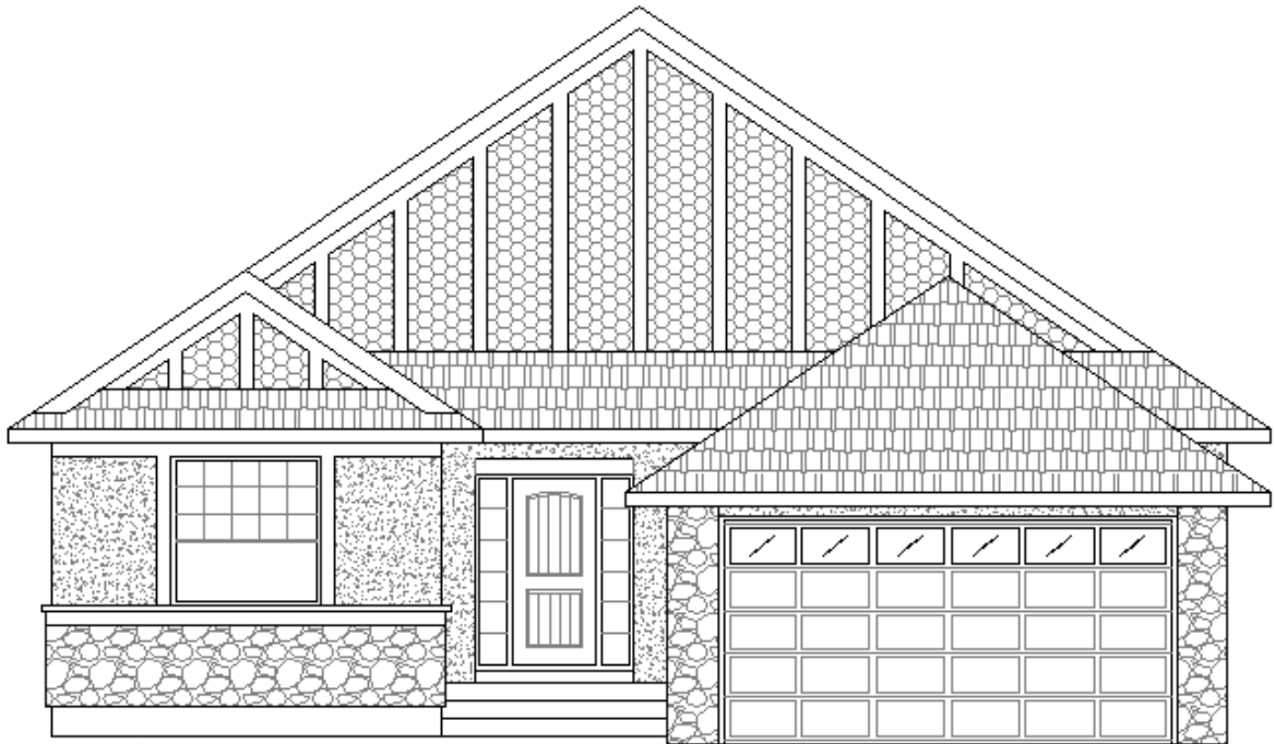
ELEVATION A
